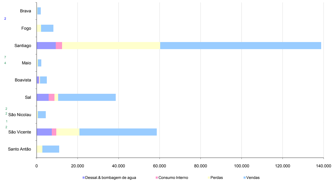
Balço da energia produzida, por ilha - 2007 (MWh/Ano)
