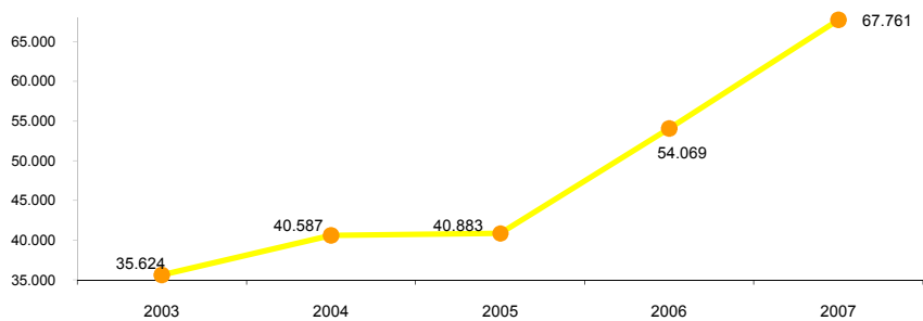
Evolução da energia utilizada para desalinização e bombagem de água, MWh
