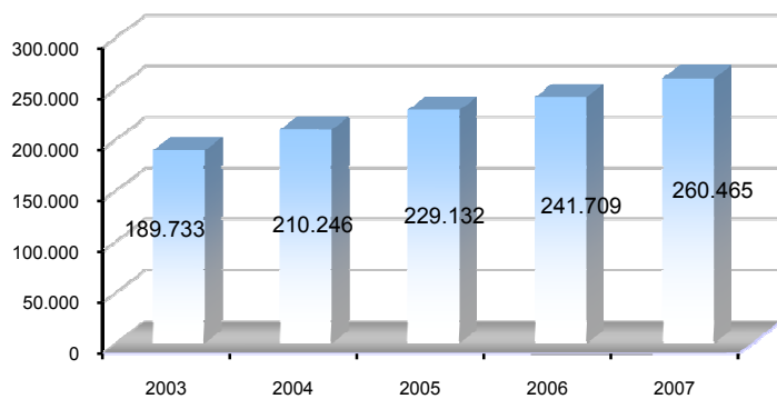
Evolução da produção de energia termica, MWh
